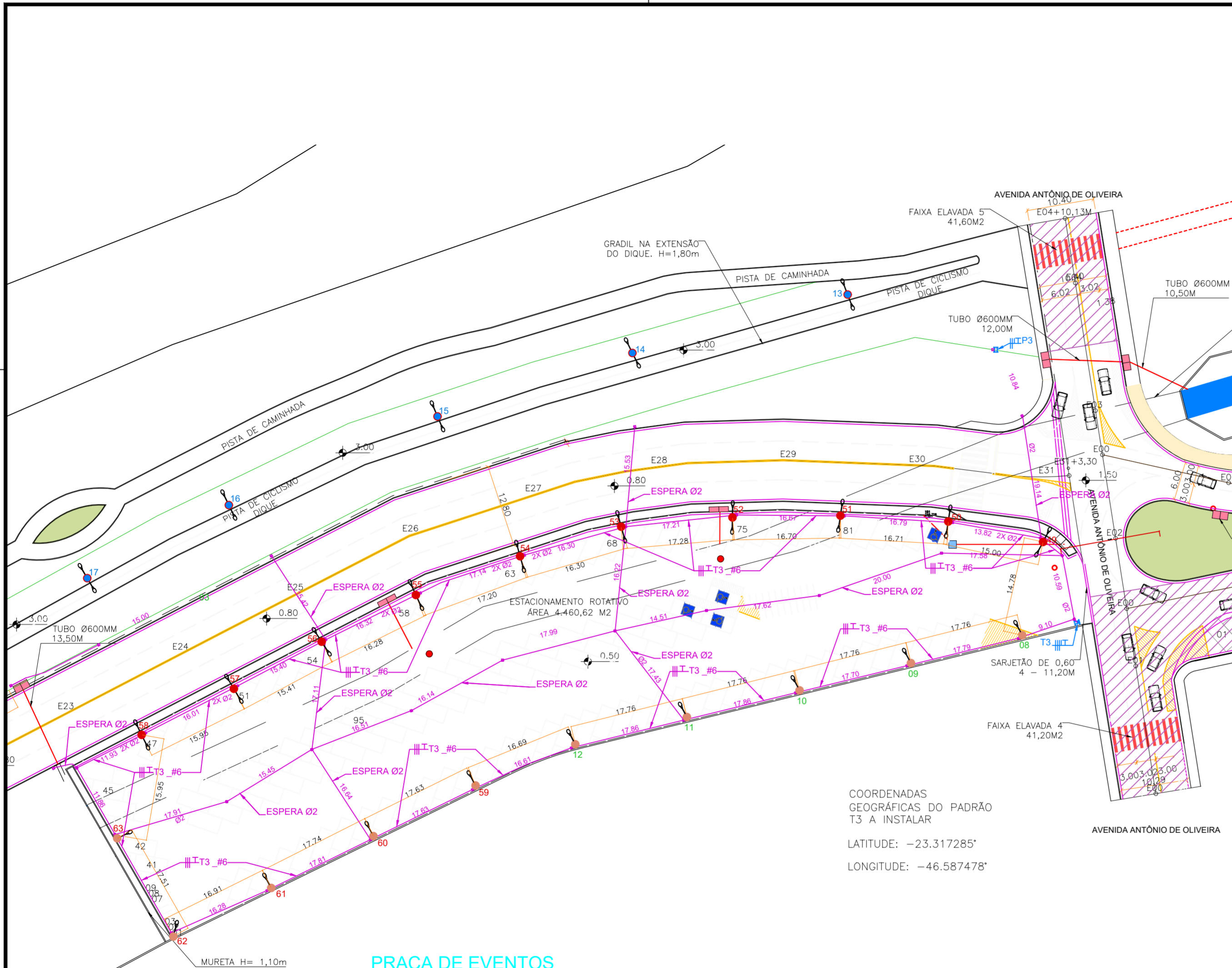
PLANTA DE ELÉTRICA esc. 1:500
